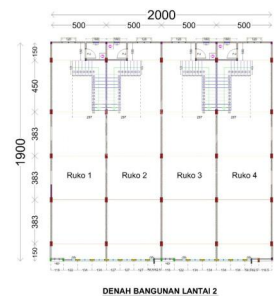
DENAH BANGUNAN LANTAI 2
