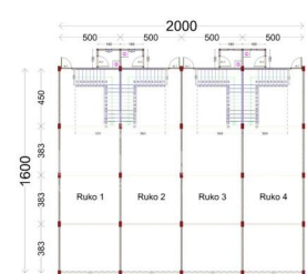
DENAH BANGUNAN LANTAI 1
